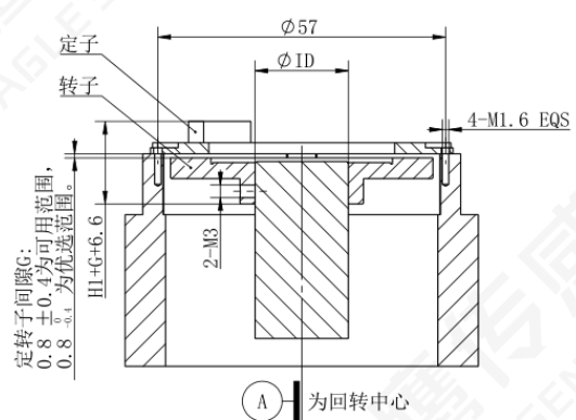
径向安装:
