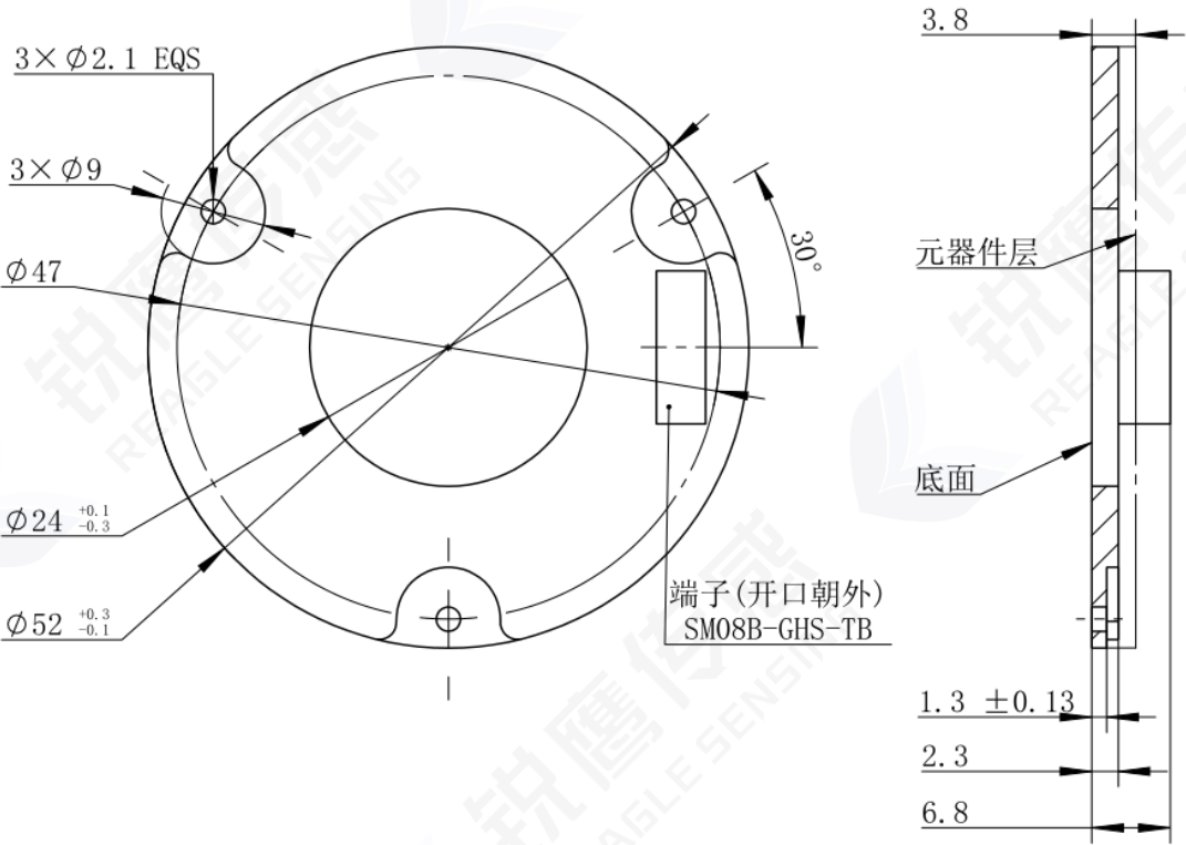
◇ 定子结构尺寸图
