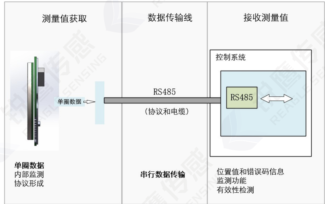
带 RS485 通讯编码器
